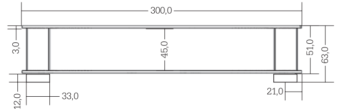
Ansicht von vorne - Maße in mm
