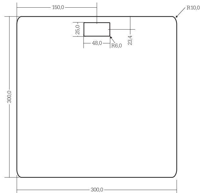
Ansicht von oben - Maße in mm
